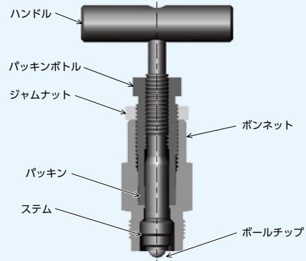
大型ボンネットストップバルブ
