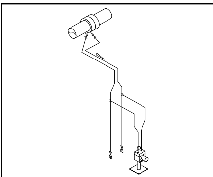
フロアー配管ラインモデル
